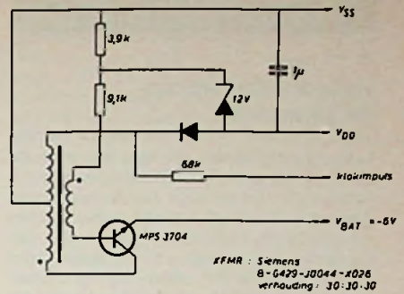
Fig. 3. Gecombineerde voedingsbron en klokimpuls-generator.
